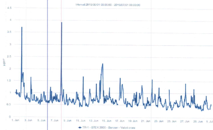
Fig. 1.5 - Benzen (µg/m 3 ) - iunie 2019
