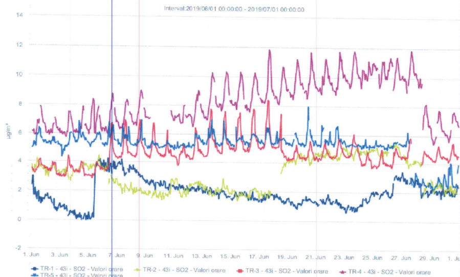
Fig. 1.1 - SO 2 ( \mu\text{g}/\text{m}^3 ) - iunie 2019
