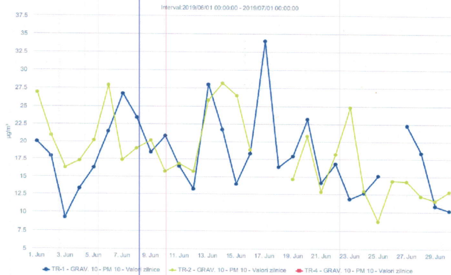
Fig. 1.6 - PM10 gravm. (µg/m 3 ) - iunie 2019
