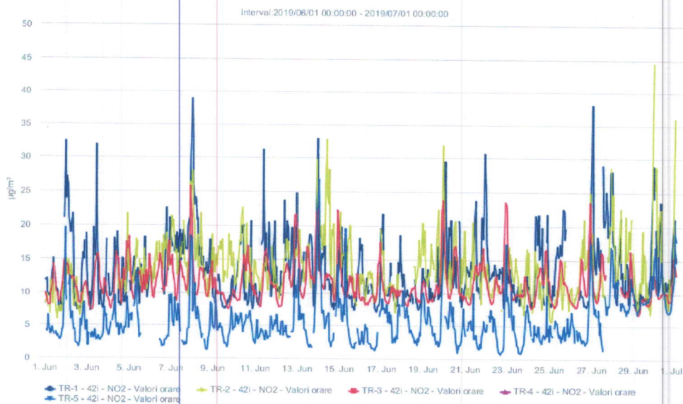
Fig. 1.2 - NO 2 ( \mu\text{g}/\text{m}^3 ) - iunie 2019
