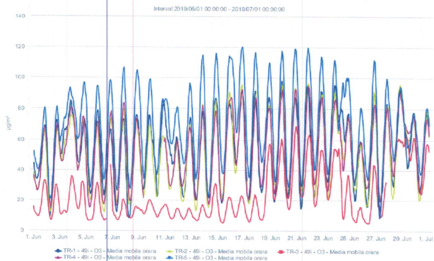
Fig. 1.3 - O 3 ( \mu\text{g}/\text{m}^3 ) - iunie 2019
