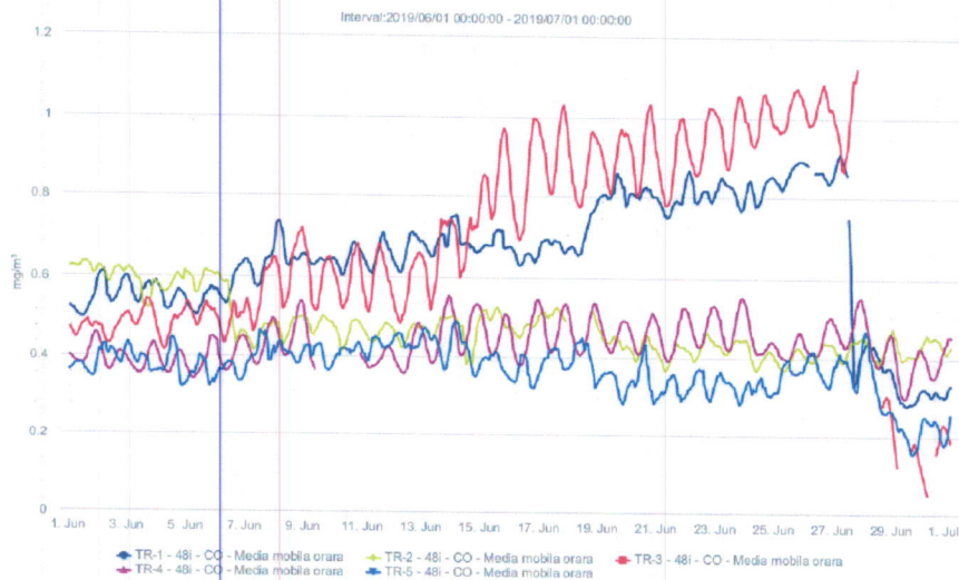
Fig. 1.4 - CO (mg/m 3 ) - iunie 2019
