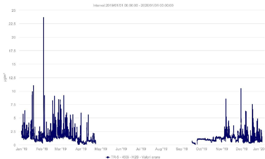
Fig. 5 Evoluția H2S în anul 2019 (concentrații medii orare)
