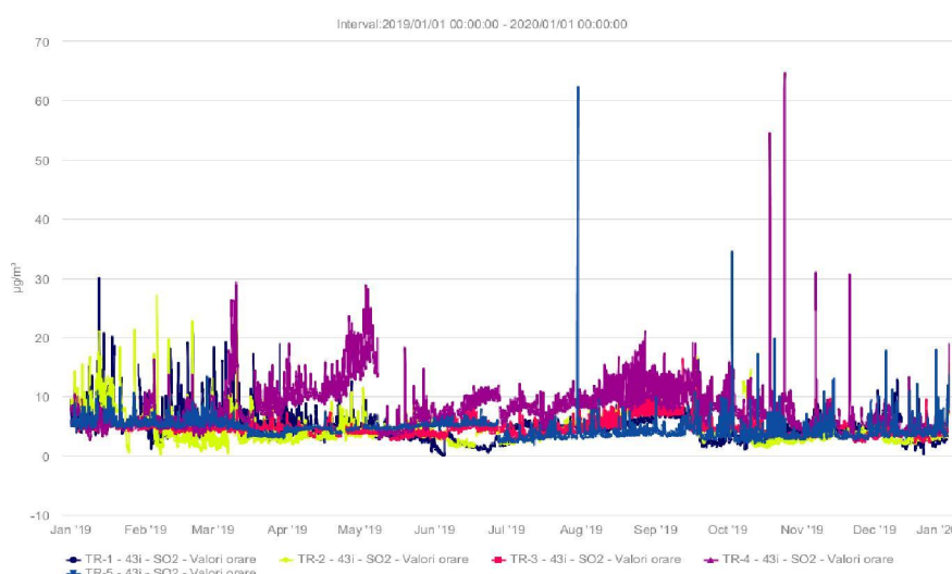
Fig. 1 Evoluția SO 2 în anul 2019 (concentrații medii orare)
