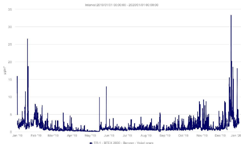
Fig. 6 Evoluția benzenului în anul 2019 (concentrații medii orare)
