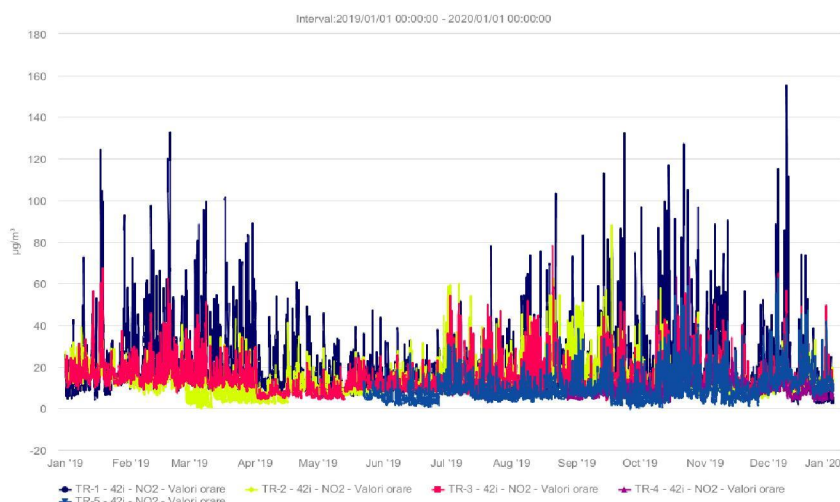
Fig. 2 Evoluția NO 2 în anul 2019 (concentrații medii orare)
