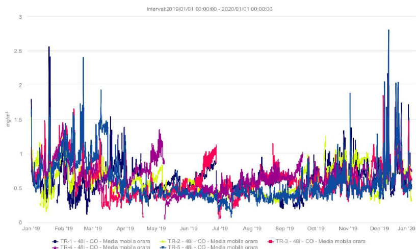
Fig. 3 Evoluția CO în anul 2019 (concentrații medii mobile)
