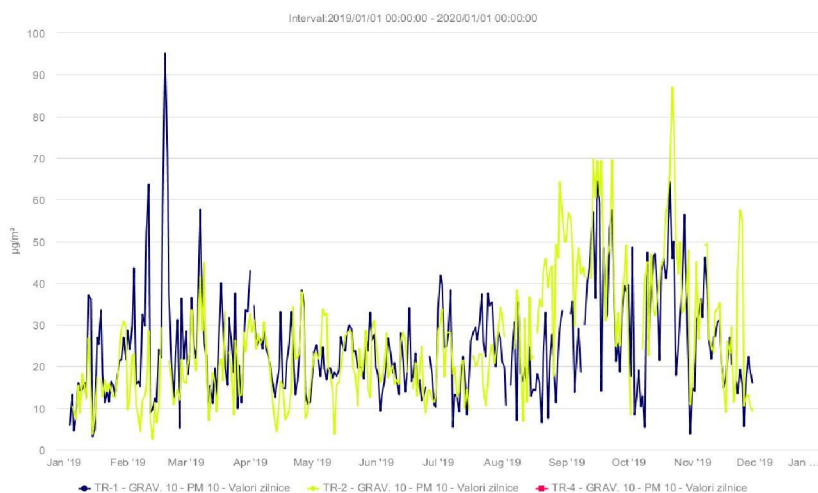
Fig. 7 Evoluția PM10 în anul 2019 (concentrații medii zilnice)
