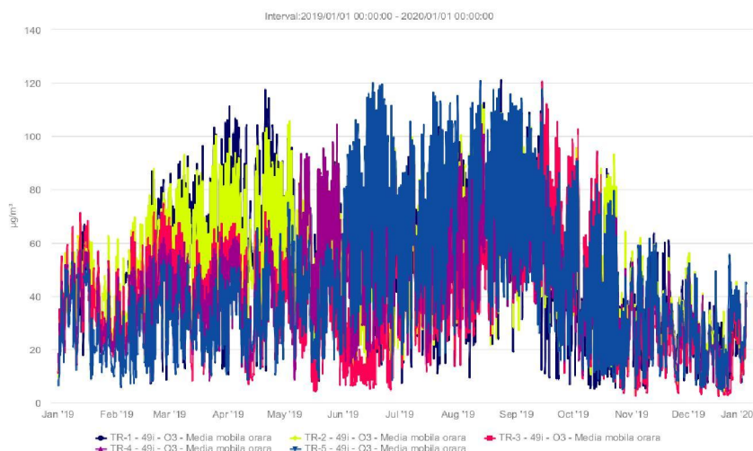
Fig. 4 Evoluția O3 în anul 2019 (concentrații medii mobile)
